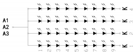
LCD 电路图
